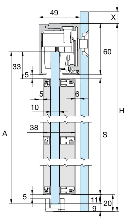
Montaje a pared de vidrio
