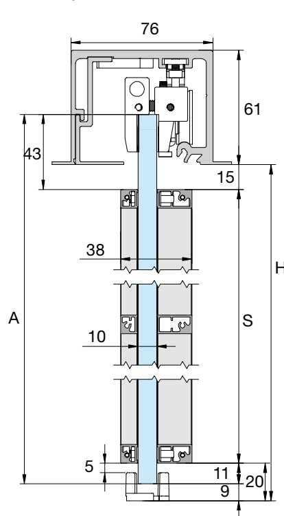
Montaje a falso techo
