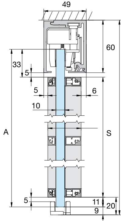
Montaje a techo
