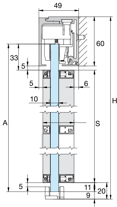
Montaje a pared
